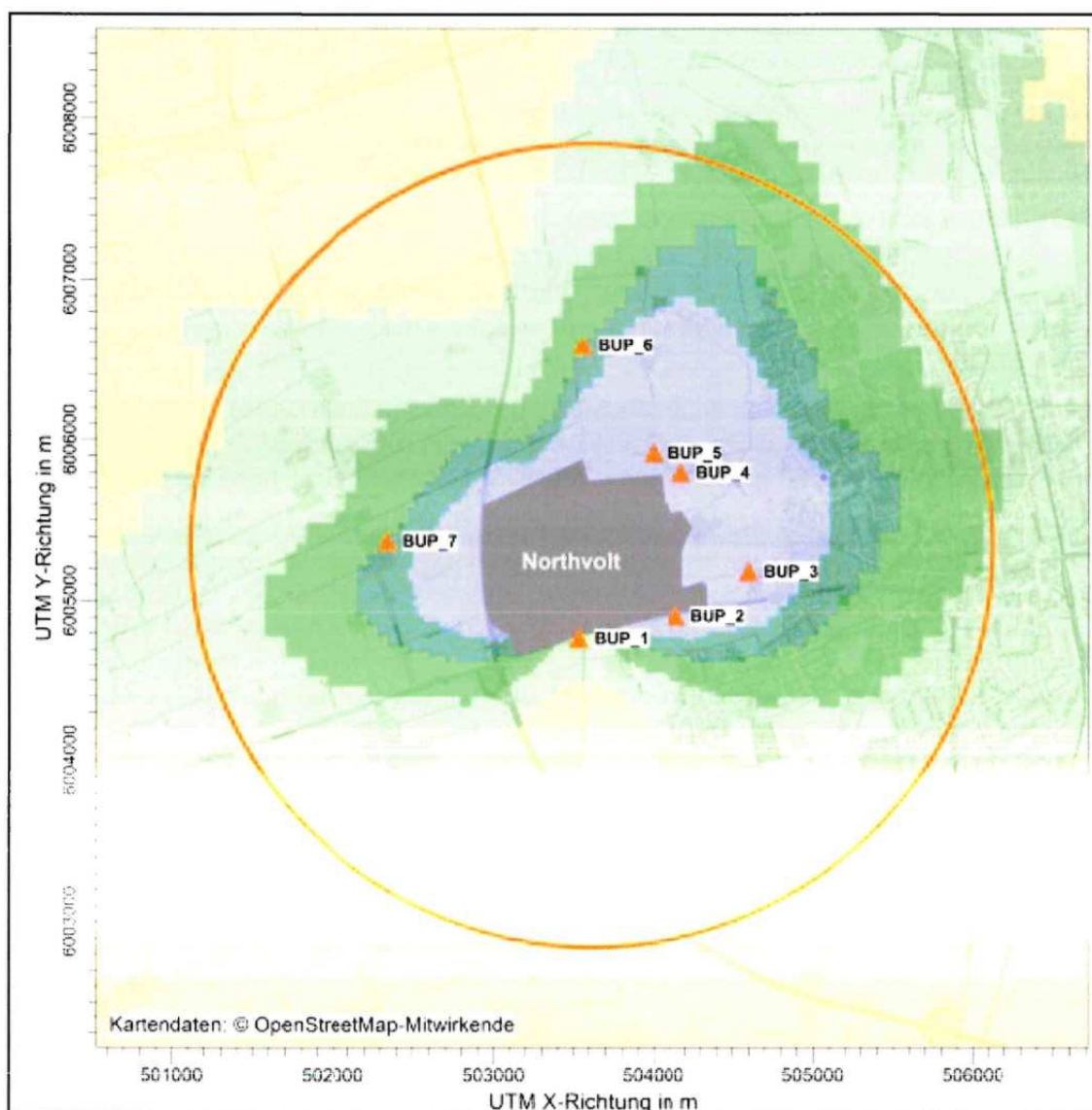
Abbildung 22: Ausbreitungsrechnung Fluorwasserstoff (GfBU 2023b)
