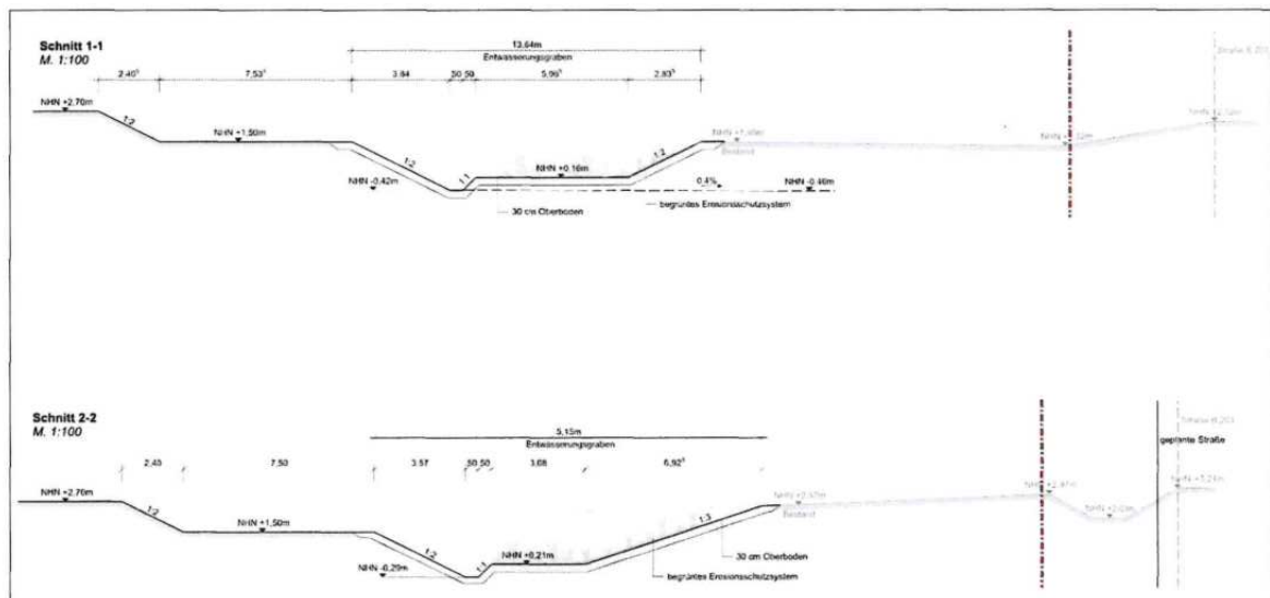
Abb.: Schemaschnitte mit alternierenden Böschungsneigungen durch den Entwässerungsgraben an der B 203 (Quelle: Entwässerungskonzept – Sellhorn, 15.08.2023)
