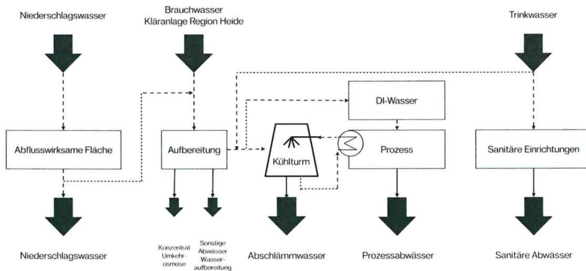
Abbildung 18: Übersicht über die Wasserflüsse in der Batteriezzellfabrik Heide (Quelle der Abbildung: Northvolt 2023)
