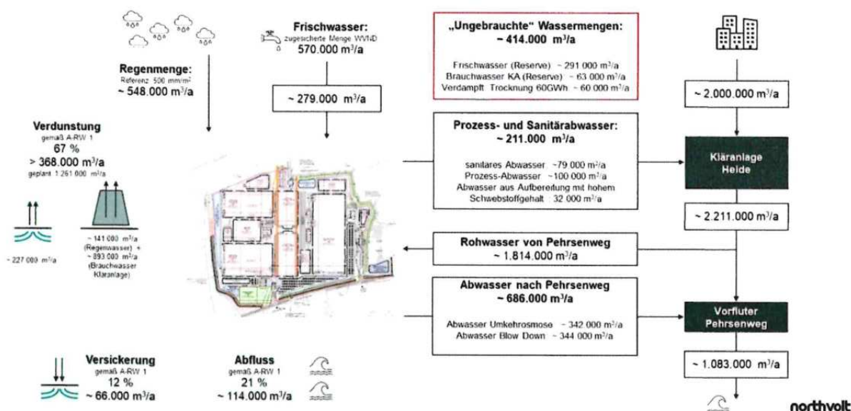
Abbildung 20: Wasserbilanz der Batteriezzellfabrik in einem „Trockenjahr“ (Quelle der Abbildung: Northvolt 2023, Zahlen auf Tausender gerundet)
